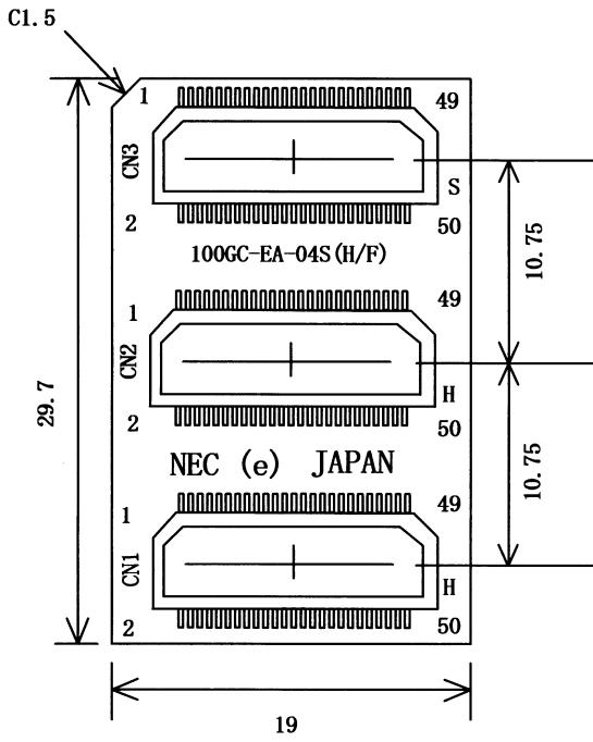
部品面寸法 (対面図)
