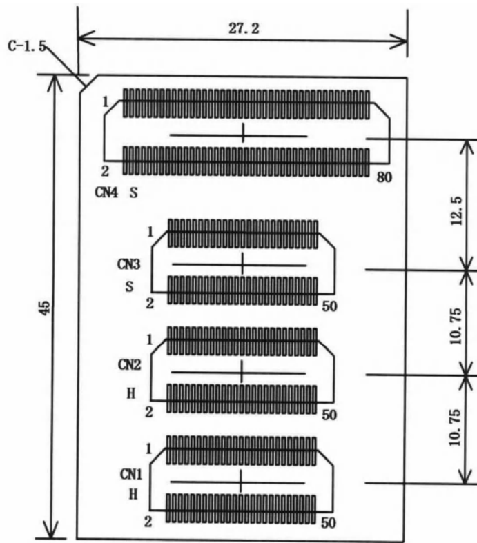
部品面寸法
