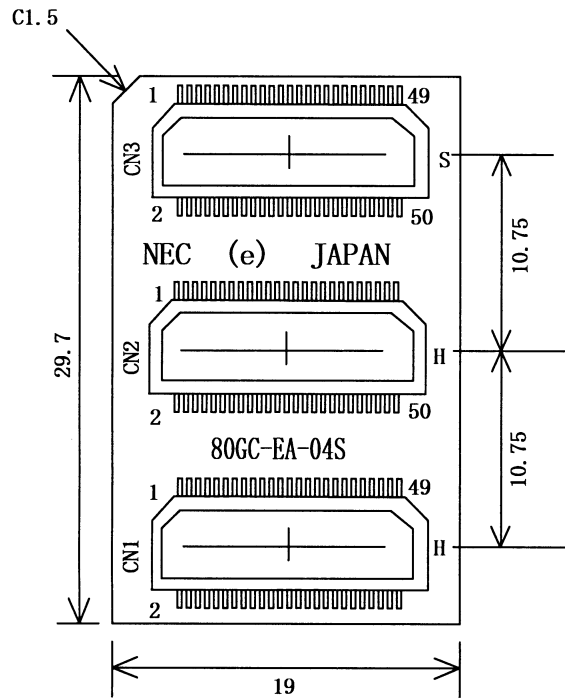
半田面寸法 (対面図)
