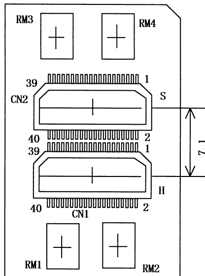
半田面寸法 (対面図)
