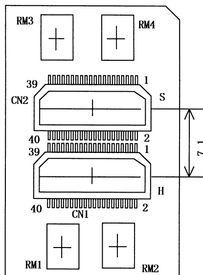
半田面寸法 (対面図)
