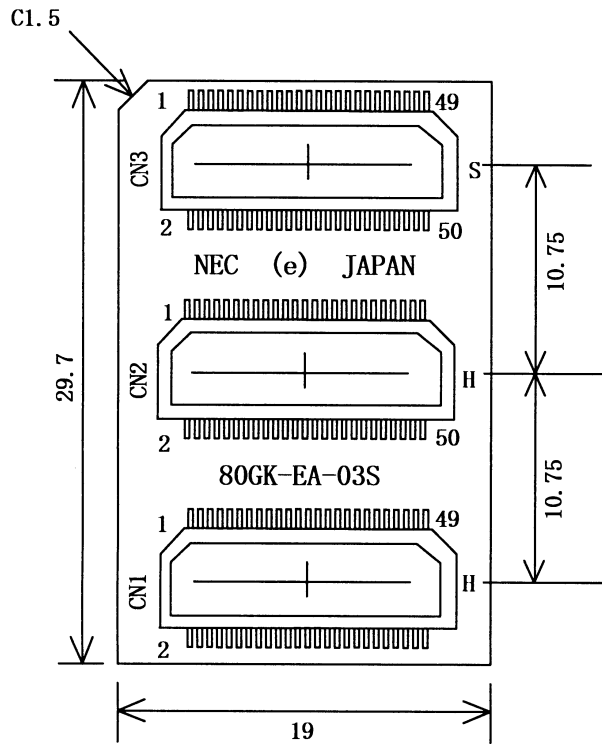
部品面寸法 (対面図)
